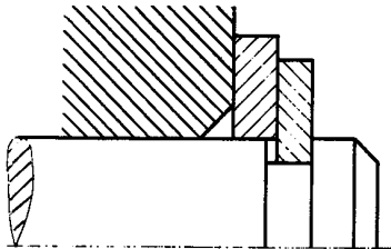
Bild 9: Seeger-Stützscheibe zwischen Seeger-Ring und Maschinenteil
