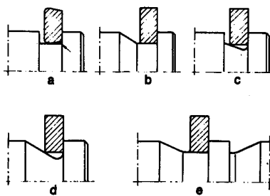
Bild 12: Nutform
