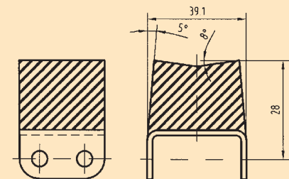
Profil Nr 1870
