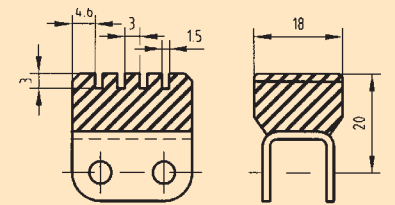
Profil Nr 4680
