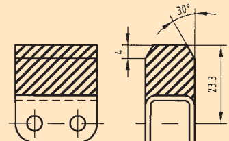
Profil Nr 1870
