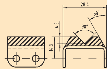
Profil Nr 0910
