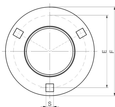
Oprawa typu „P”
