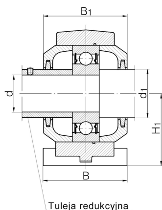
Oprawa TSP ...
