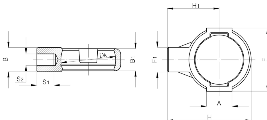
Wymiary opraw naciagowych typu SPK
