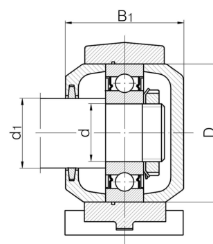
Oprawa TSN ...
