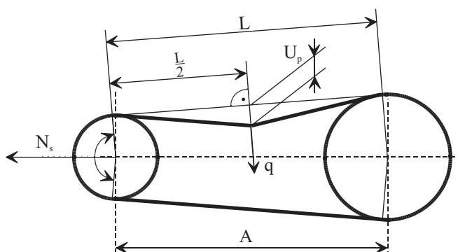
Rys. 5.1. Kontrola naciągu pasa przez pomiar ugięcia cięzna pasa
