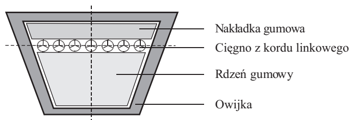
Rys. 2.3. Budowa pasa normalnoprofilowego (klasycznego)
